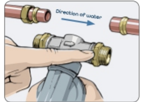
5. Paigalda surverõngad ja ühendusmuhv
